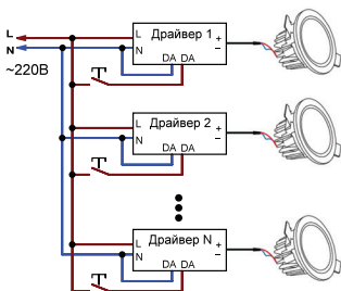
Рис.2. Структурная схема подключения оборудования при использовании кнопки Touch DIM
