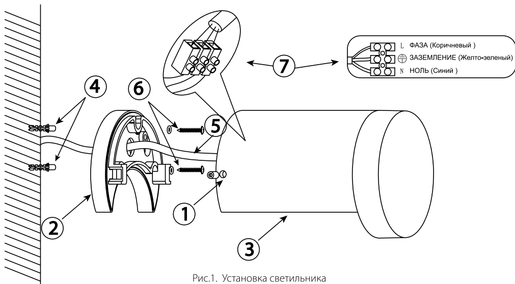
Рис.1. Установка светильника
