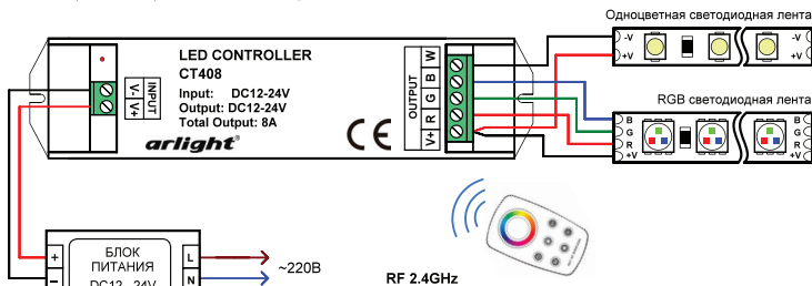
Рис.1. Подключение RGBW контроллера CT408. К контроллеру CT309 подключается только RGB светодиодная лента.
